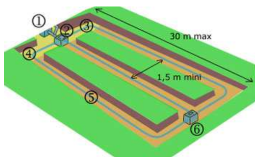
Principe général de l'épandage souterrain 3
