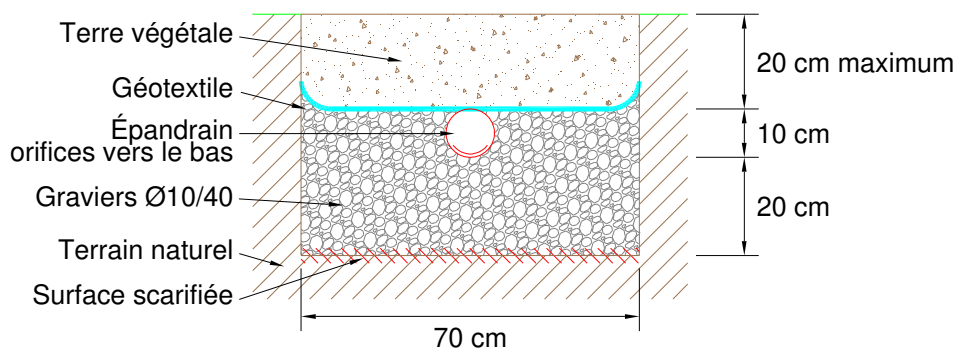
Coupe transversale d'une tranchée d'infiltration - Généralités
